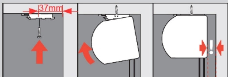
Deckenmontage
