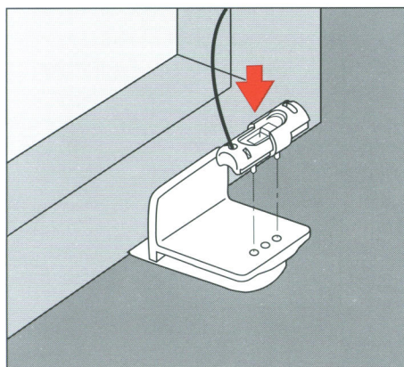
Cosiflor F mit Pendelsicherung Cosiflor F with guide wire Cosiflor F koordrem en koordgeleiding Cosiflor F avec immobilisation Cosiflor F с фиксацией отката
